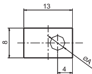
Style 056: A=\varnothing 4.2 Style 056-1: A=\varnothing 5.2
