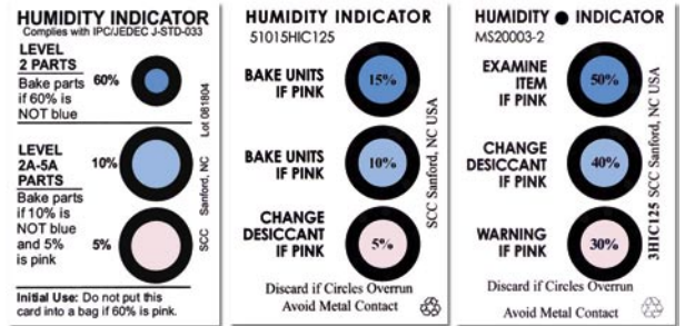
kosteusindikaattori-kortti 5, 10, 60% RH
